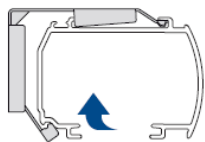
Höjd: 37 mm inkl fäste Djup: 52 mm inkl fäste
