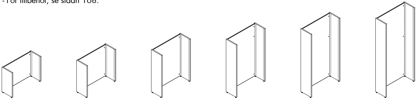
Enkelsidig fristående sektion - H720/920/1220/1520/1820/2120 mm
