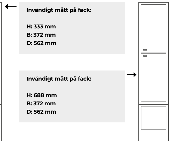
PDF4/19-2 1932 X 410 X 580
