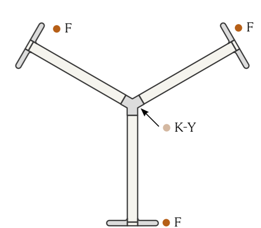
EXEMPEL (Koppling Y-120°)
