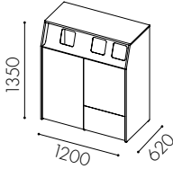
W3515 Hel dörr till vänster för rullkär 140 l *, dörr ovan till för 2x60 kär och lådutdrag undertill till höger **
