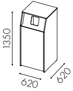
W3510 Hel dörr för rullkär 140 liter *
